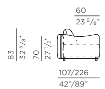
larghezza bracciolo 21 cm armrest width 8 1/4"
